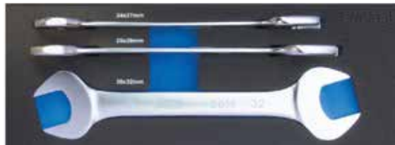
MOD. 1805 B STEEKSLEUTELS VAN 24 TOT 32MM 3 DELIG
